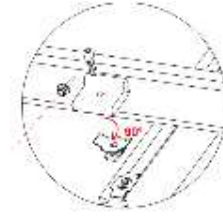
Dispositif anti-glissement pour le climber 63
